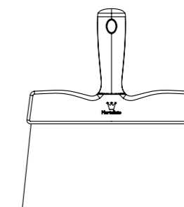
50RAS07 Total size: 225x200 mm Handle: h 130x189,7 mm Lama - Blade 200 x h 95 mm
